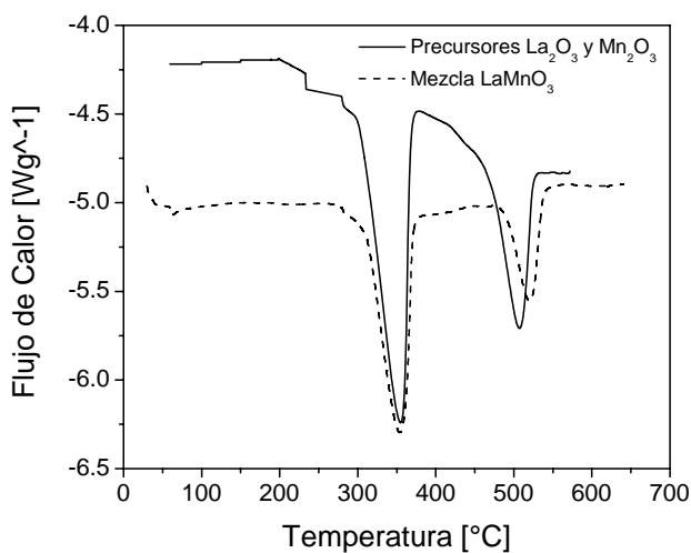
Figura 2. DSC de la manganita de lantano mediante el método cerámico.
