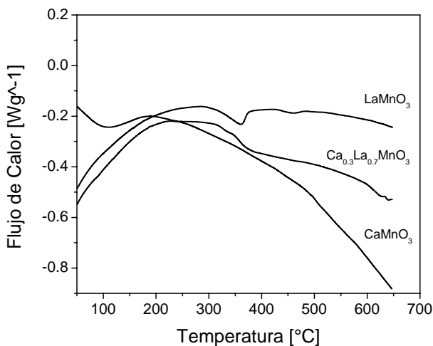
Figura 11. DSC de manganitas con diferentes niveles de dopaje a 4.5 horas de molienda.
